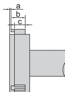
C型 50-300mm, 硬质合金测量面
